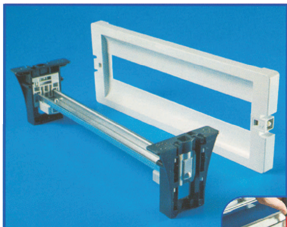
Jednoduchá montáž DIN lišt - zaistenie pomocou skrutkovača
