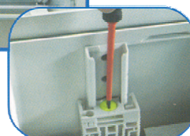
Montážnu dosku je možné ukotviť pomocou posuvných zámkov
