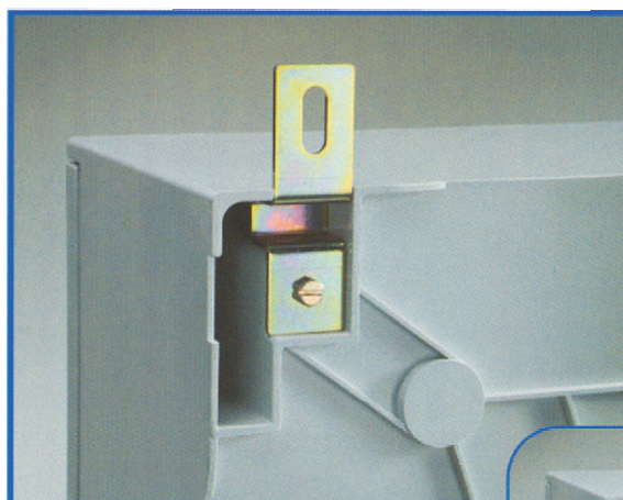
Záves je možné osadiť horizontálne i vertikálne. Na objednávku aj nerezový.
